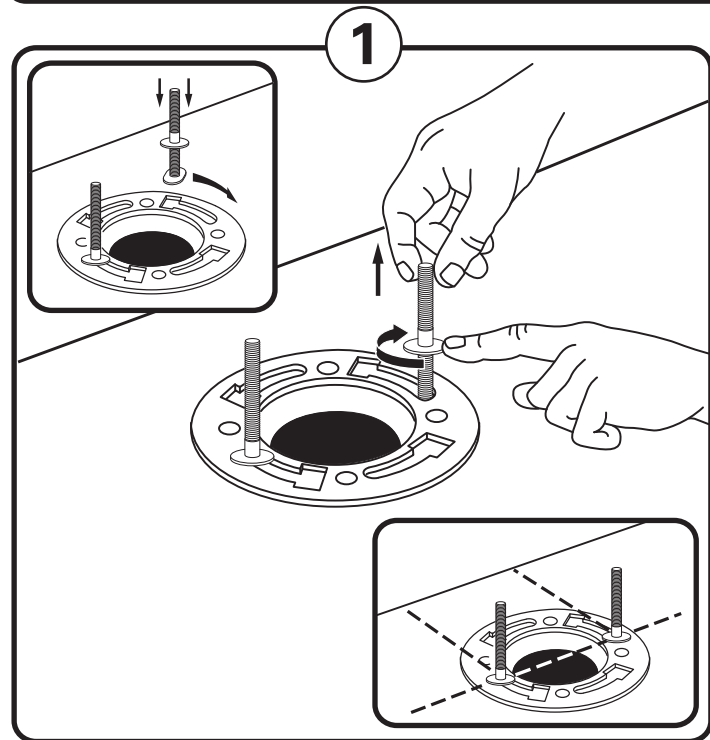
Recommended fitting type for back-to-back installations. Type de raccord recommandé pour les installations face à face.
