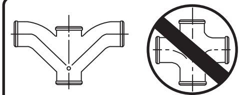
Recommended fitting type for back-to-back installations. Type de raccord recommandé pour les installations face à face.
